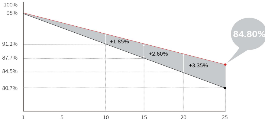
质保曲线图
